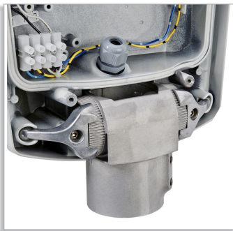
Regulowany zaczepek montażowy
