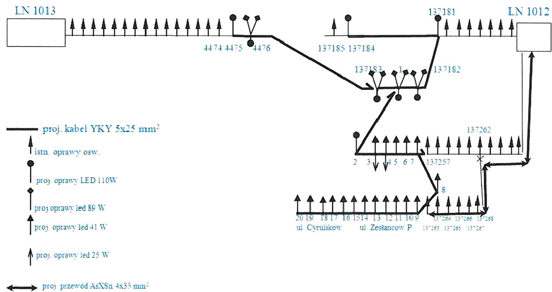
Rys. nr 2 Schemat ideowy oświetlenia ul. Zesłańców Polskich i Cyrulików w Warszawie
